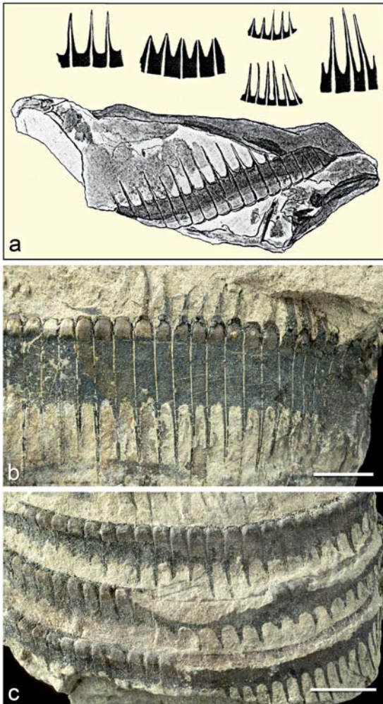
Abb. 5.6 Die pflanzentaphonomische Entzifferung der angeblichen Mittelnaht bei Equisetites -Blattsitzen. a Oben: Blattspitzen von Equisetites laevis ; aus HARRIS (1931), Abb. 3 a-e. a Unten: „ Equisetites cuspidatus “ (= E. arenaceus ), Sinsheim (aus STERNBERG 1820–1838: Taf. 31, Fig. 8). b Equisetites arenaceus , Blattscheide, sowohl mit teilweise erhaltenen Blattspitzen als auch den an den Rändern herabreichenden Kommissuralfurchen. SCHL-048. c E. arenaceus , ineinander steckende Blattscheiden mit verdickt erscheinenden dreidimensional-kuppelförmigen Blattspitzen und arkadenartig geschwungenen Rändern der Segmente, hervorgerufen durch die teilweise erhaltenen Randpartien an den Kanten der Kommissuralfurchen. SCHL-167.
