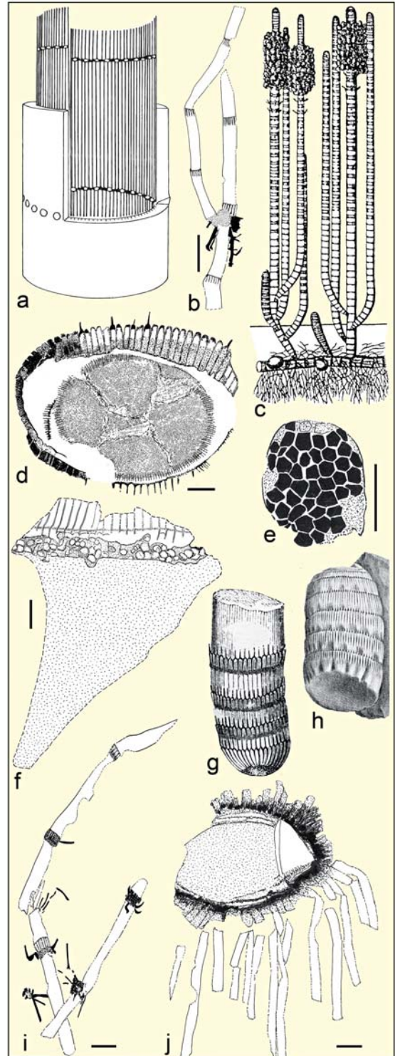
Abb. 5.12 Umgezeichnete Details sowie Rekonstruktion des Schachtelhalms Equisetites arenaceus . Maßstab jeweils 1 cm. a Schemazeichnung zur Entstehung von gerieften Gefäßbündel-Steinkernen. Nach Weber (1968), verändert. b Sich gabelnde Seitenachse, mit Adventivwurzel. SCHL-883a. c Lebensbild, nach Frentzen (1934). d Diaphragma (Knotenscheidewand), noch in organischer Verbindung mit der Blattscheide. SCHL-804. e Sporophyllstand, mit polygonalem Umriß der Sporophylle. SCHL-047. f Mehrzeilige Astnarben an einem Nodium. SCHL-826a. g Rekonstruktion der basalen Sprossachse. Nach Heer, aus Kelber (2009). h Architektur des Sprossgipfelbereichs. Aus Schoenlein (1865). i Isolierte Seitenachsen mit Adventivwurzeln. SCHL-842. j Schrägansicht eines Diaphragmas, teilweise noch mit dünnen Zweigen in organischer Verbindung. SCHL-895.
