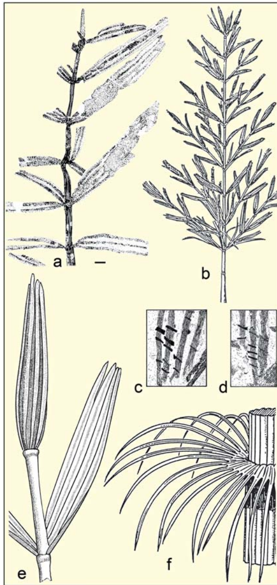
Abb. 5.18 Die Schachtelhalm-Gattungen Schizoneura und Phyllothea . a Schizoneura paradoxa , beblätterte Achse; SCHL-060. Maßstab 1 cm. b Schizoneura paradoxa , Rekonstruktionsversuch (verändert nach MÄGDEFRAU 1968). c, d Transversale, riegelartige Strukturen an Schizoneura -Blättern. Über die Ursache dieser Bildungen ist noch nichts Näheres bekannt. Detail, SCHL-059 (aus KELBER 1983: Taf. 4f). e Rekonstruktion einer beblätterten Achse von Schizoneura paradoxa . An den Knotenzonen entspringen gegenständige Blatteinheiten. Die Blattlappen können sich später in schmale Einzelblätter zerteilen (umgezeichnet nach SCHIMPER 1869–1874). f Phyllothea equisetoides als Beispiel für die Architektur der Phyllothea -Pflanze aus dem Lettenkeuper (aus BOUREAU 1964).
