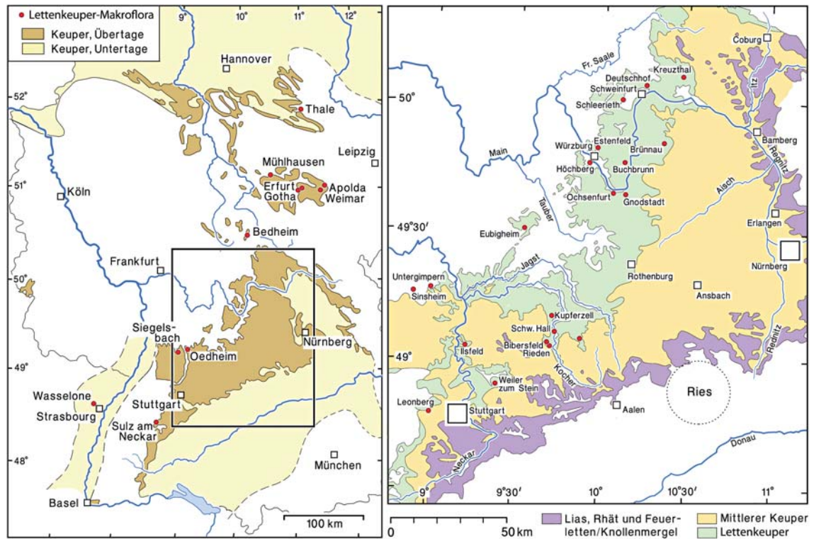
Abb. 5.1 Makroflora-Fundpunkte aus dem Lettenkeuper. Geologie teilweise nach BEUTLER (1998), verändert.
