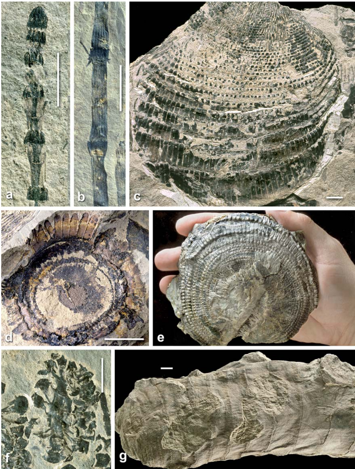
Abb. 5.11 Sprossgipfel, Sporophyllstand, Diaphragma, Rhizom, Astabgänge und Seitenachsen des Schachtelhalms Equisetites arenaceus . Maßstab jeweils 1 cm. a Distales Ende einer schmalen Seitenachse. SCHL-844a. b Seitenachse von Equisetites arenaeus mit Adventivwurzeln an den Nodien. SCHL-796. c Sproßgipfelbereich, mit teleskopartig ineinander steckenden Internodien. SCHL-040. d Diaphragma, Blattscheide und radial angelegte Astabgänge. SCHL-812a; e Sproßgipfel, Draufsicht, OCH-007a. f Sporophyllstand, Seitenansicht, SCHL-062a; g Erdsproß (Rhizom), erhalten als Rindensteinkern, HÖCH-008.
