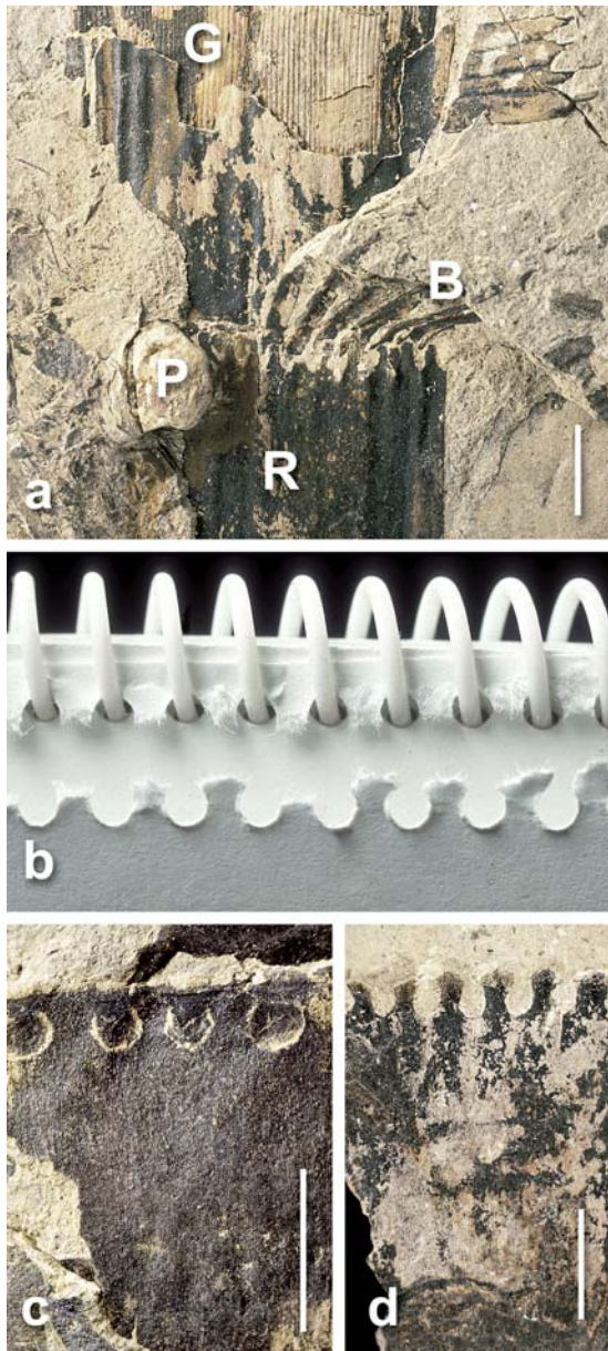
Abb. 5.5 Die Bildung der pflanzen-taphonomischen Zerreibungsmuster an der Rinde des Schachtelhalmes Neocalamites merianii , die sogenannten „terminalen Nodialläppchen“ ( sensu ROSELT 1954). a Beblättertes Achsenfragment. Der flach ellipsoide Steinkern zeigt die Abdrücke der Gefäßbündel (G) und die flachgewellte Rinde (R) mit den wirtelig angeordneten Austrittsstellen der schmal ausgezogenen Blätter (B) in organischer Verbindung. Links: eine ehemalige Pyritkonkretion (P), jetzt in Goethit umgewandelt. SCHL-1067. b Die Ausreißkanten an einem Spiralblock, zum Verständnis des pflanzen-taphonomischen Vorgangs. c Isolierte Rindenhaut mit noch nahezu unverletzten Blatt-Austrittsstellen. SCHL-2004-2. d Rindenfragment mit den kennzeichnenden terminalen Nodialläppchen. Kleinste Rindenfragmente können durch dieses Merkmal der N. merianii -Pflanze zugeordnet werden. SCHL-2004-3.
