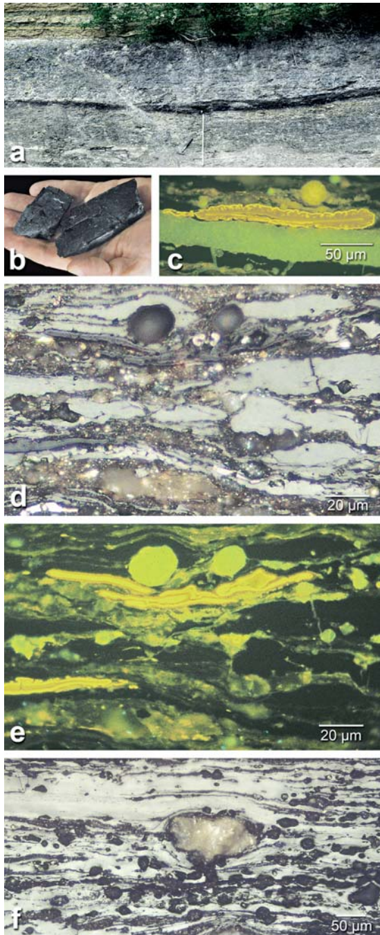
Abb. 5.3 Makro- und mikroskopische Ansicht der Lettenkohle aus dem Lettenkeuper. Präparatherstellung, Mikrofotos und Definition der Kohlenmazerale (Abb. 5.3c-f) von B. LIGOUIS, LAOP Tübingen. a Geringmächtige Kohlenlinse, maximal 35 cm mächtig, nach links auskeilend. Werksandsteinbruch Schleierieth. Im oberen Bildteil die beigefarbenen basalen Kalke der Albertibank. Aufnahme von 2006, Maßstab: Zollstock 1 m bzw. Geologenhämmer, Bildmitte unten. b Die Lettenkohle aus der Schleieriether Kohlenlinse im Handstück. Die bläulich-tiefschwarz bis stumpf-anthrazit gefärbten Kohlenproben sind aufgrund tektonischer Vorgänge durch messerscharfe Klüfflflächen gekennzeichnet. c Polierter Kohlenanschliff der Schleieriether Lettenkohle. Fluoreszenzmikroskopie, Öl-Immersion. Der Querschnitt durch eine gelblich-orange fluoreszierende und ornamentierte Makrospore (Sporinit) in der Bildmitte. Darüber (nicht im gleichen Schärfenbereich) eine rundliche Karbonatkonkretion. d Polierter Kohlenanschliff der Schleieriether Lettenkohle. Öl-Immersion. Die Vitrinit-Mazerale Collotelinit und Collodetrinit sind mittelgrau gefärbt, im oberen Bildbereich befinden sich einige Quarzkörner (nahezu in Schwarz). Am unteren Bildrand langgestreckte körnig hellbraune Karbonataggregate. Kleine hell-gelblich reflektierende Körner, oft mit überstrahlenden unscharfen Rändern, sind Pyritframboide. Die dunkleren Bildpartien bestehen vorwiegend aus Tonmineralen, unter denen sich auch Aggregate von Sporinit, Kutinit oder Liptodetrinit verborgen haben können. e Polierter Kohlenanschliff der Schleieriether Lettenkohle, gleicher Bildausschnitt wie Abb. 5.3d. Fluoreszenzmikroskopie, Öl-Immersion. Gelblich-orange fluoreszierende Sporinit-Aggregate, darüber (nicht im gleichen Schärfenbereich) zwei rundlich geformte Quarze. f Polierter Kohlenanschliff, Öl-Immersion. Zahlreiche gerundete Quarzkörner, eingebettet in den Vitrinit-Mazerale Collotelinit und Collodetrinit (grau). Im mittleren Bildteil eine größere Karbonatkonkretion, körnig, hellbraun). Die dunklen Bildteile bestehen vorwiegend aus Tonmineralen, in denen sich auch vereinzelt Aggregate von Sporinit, Kutinit und Liptodetrinit verbergen können. Diese sind jedoch nur durch Fluoreszenzbeleuchtung deutlicher erkennbar (vgl. Abb. 5.3c, e).
