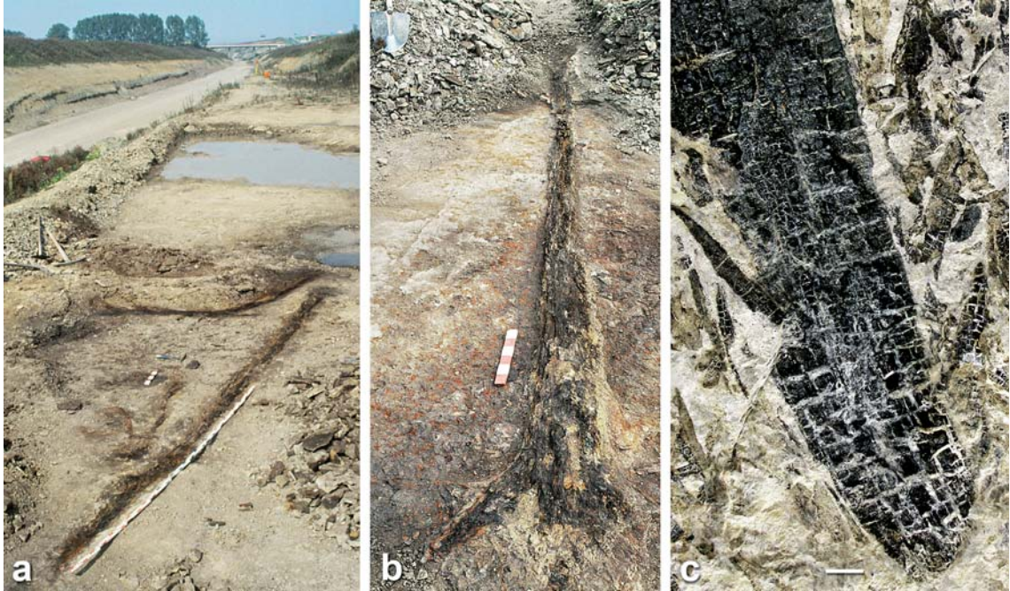
Abb. 5.4 Verdriftete Holzfossilien in Pseudogagat-Erhaltung aus dem Lettenkeuper. a Schichtfläche mit mehreren subparallel eingelegten Baumstämmen. Lettenkeuper, ICE-Trasse südlich der BAB 71-Ausfahrt Arnstadt-Süd. Grabung des Naturhistorischen Museums Schleusingen. Foto R. WERNEBURG, aus WERNEBURG (2004). b Detail aus Abb. 5.4a. Freigelegter Baumstamm von mehr als 6 m Länge, vorwiegend in Pseudogagat-Erhaltung, mit rudimentärem Wurzelteller. Foto R. WERNEBURG, aus WERNEBURG (2004). c Inkohltes Treibholz in Pseudogagat-Erhaltung, mit transversalen Schwundrissen. Grenz dolomit (Lettenkeuper), Prichsenstadt, Kanalbau Nähe Bahnhof. Sammlung K.-P. KELBER, Würzburg.
