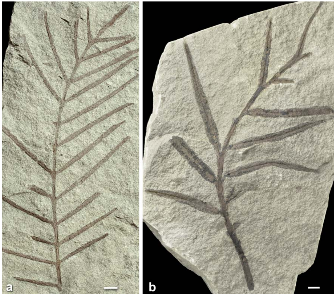
Abb. 5.23 Wedel von Samenfarne in Sandsteinerhaltung aus dem Lettenkeuper. Maßstab: 1 cm. a „ Selenocarpidium gracillimum SANDBERGER“. Estenfeld, PIW F3733. b Wedel von Scytophyllum bergeri , vormals als „ Cycadites rumpfi “ bezeichnet. Aus der ehemaligen Sammlung von FRIEDRICH v. ALBERTI (Original zu SCHIMPER 1869–1874). SMNS P.697/7.
