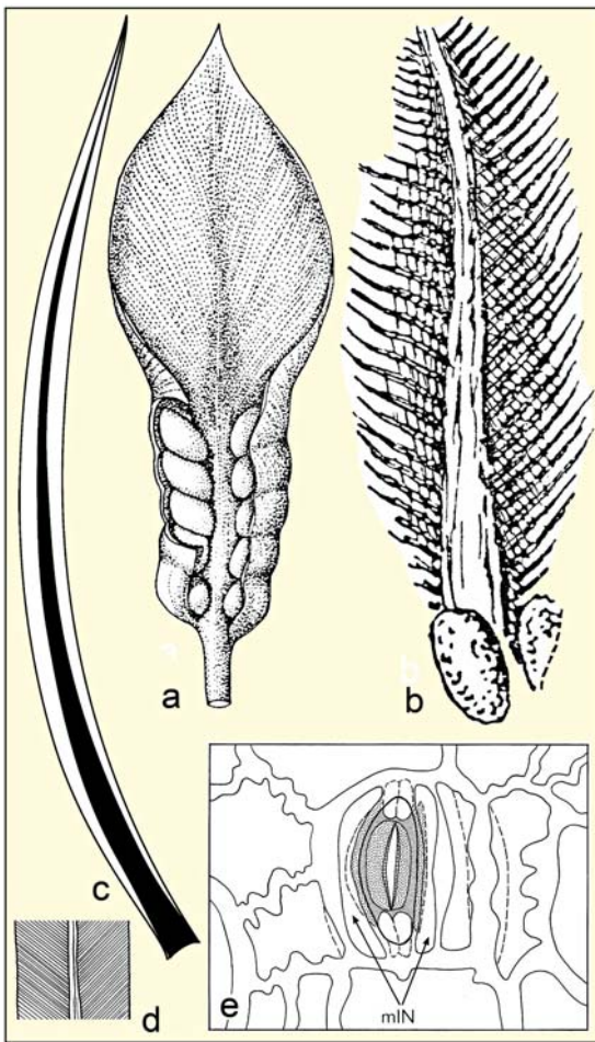
Abb. 5.25 Cycadeen-Fruchtifikationen, die Formgattung Taeniopteris und der Bau der Spaltöffnungsapparate bei den Bennettiteen. a Archaeocycas , ein altertümliches Cycadeen-Fruchtblatt aus dem Perm (aus MAMAY 1969). Das auf Abb. 5.24d abgebildete Exemplar aus dem Lettenkeuper ähnelt mit seinem basalen Bereich Archaeocycas , die distale Partie des Fruchtblattes ist jedoch genauso gefiedert wie Dioonitocarpidium pennaeforme . b Dioonitocarpidium pennaeforme , Skizze eines Fruchtblattes mit paarweisen gekörnelten Samen an der Basis. Wahrscheinlich identisch mit den Pflanzenabdruck in Abb. 5.24g, i (Zeichnung aus COMPTER 1922, Taf. 3, Fig. 40). c Taeniopteris kelberi , schematisierte Blattgestalt (aus KELBER 2009). Rekonstruiert nach Abb. 5.24a. d Taeniopteris kelberi , Schema der Blattnervatur. Siehe auch Abb. 5.24b. e Die syndetocheile Spaltöffnung der Bennettiteen. Aus der Mutterzelle (gepunktet) gehen außer den beiden Schließzellen noch zwei Nebenzellen hervor. mlN = mesogone laterale Nebenzellen (umgezeichnet nach FLORIN 1933).
