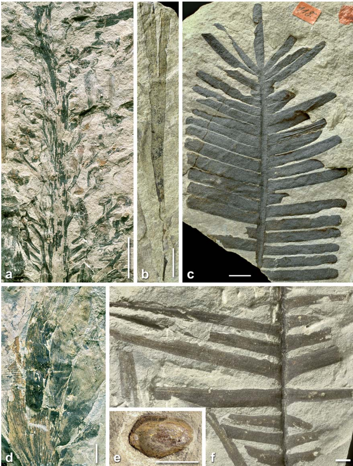
Abb. 5.26 Ginkgogewächse und Bennettiteen aus dem Lettenkeuper. Maßstab: 1 cm. a Blütenstand, gen. et sp. indet, möglicherweise zu den Ginkgophyten gehörend, SCHL-800. b Sphenobaiera sp., sich teilendes Blatt. SCHL-700a. c Pterophyllum brevipenne , Wedelspitze, Buchbrunn (Original zu SCHOENLEIN 1865, Taf. 13, Fig. 2); Nr. 1989/492, Museum für Naturkunde, Berlin. d Ginkgo sp., Blattschopf mit typischer Nervatur. SCHL-2004-9. e Carpolithus sp., fossiler Same in Roteisensteinerhaltung. GNO-20042. f Pterophyllum robustum , Wedel. Bibersfeld. SMNS P.778/15.
