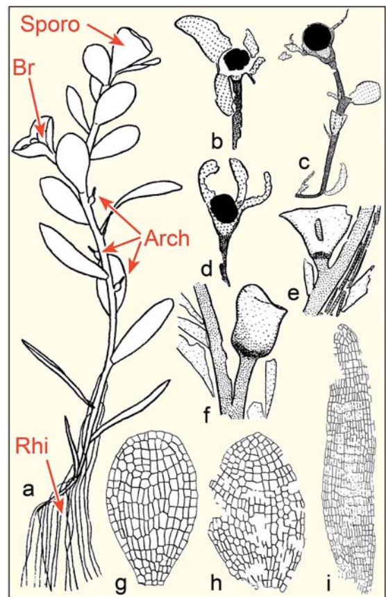
Abb. 5.28 Rekonstruktion von Naiadita lanceolata (Marchantiophyta, Bryophyta) und umgezeichnete N. lanceolata -Fossilien aus dem Rhätium von England zum Vergleich mit den Neufunden aus dem Lettenkeuper. b-i: Aus HARRIS (1938). a Naiadita lanceolata -Rekonstruktion. Achse beblättert sowohl mit eher länglichen als auch rundlich ovalen Blättchen. Sporo = Sporophyll, Br. = Brutknospenbecher (gemmae cup); Arch = Archegonien; Rhi = Rhizoide (aus HARRIS 1939). b-d Sporogone (schwarz) in situ , teilweise noch umgeben von Blättchen der Perianth-Struktur. e-f Seitlich an der Achse herausgewachsene Brutknospenbecher (gemmae cups). g-i Form und Zellstruktur einiger Blättchen.
