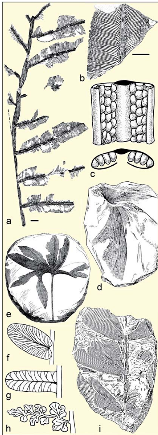
Abb. 5.20 Echte Farne und problematische farnlaubige Reste aus dem Lettenkeuper. a Wedelfragment der Marattiaceae Danaeopsis angustifolia . Maßstab 1 cm. SCHL-064a. b Fiederspitze von Danaeopsis angustifolia . Die sich gabelnden Fiedernerven wachsen am Blattrand wieder zusammen. OCH-061. c Sche-
