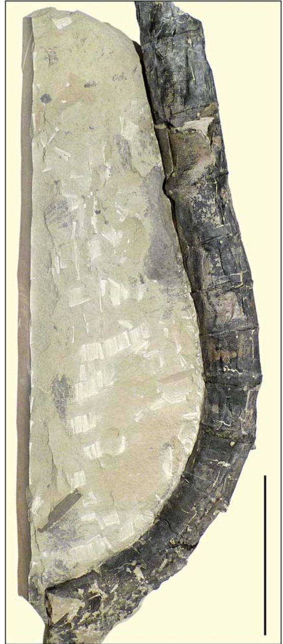
Abb. 5.10 Rhizom und basaler Spross von Equisetites arenaceus . Hauptsandstein, Steinbruch Schumann, Vellberg- Eschenau. MHI-Ku 1979. Foto H. HAGDORN, Maßstab: 50 cm.
